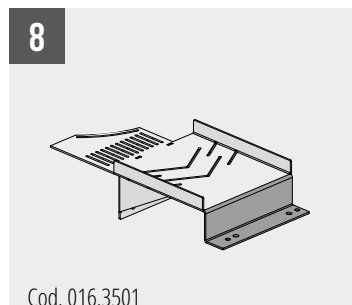
TIGER 372 CNC LR 4.0 RC - 402 CNC HR 4.0 RC Adattatore lato scarico
