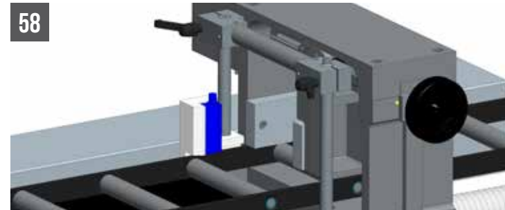
TIGER 372 CNC LR 4.0/RC - TIGER 402 CNC HR 4.0/RC Kit alimentazione progressiva continua (sistema sensori presenza barra per alimentazione progressiva automatica)
