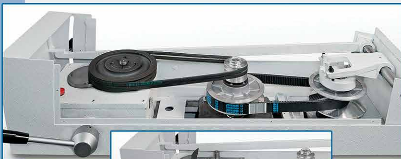
Trasmissione con variatore ritardo (VAR.R) Modd. 35/40/45 • Trasmissione con variatore ad ingranaggi • Variation des vitesses par variateur avec engrenages • Gears + belts speed variator • Getriebe Stufenlos
