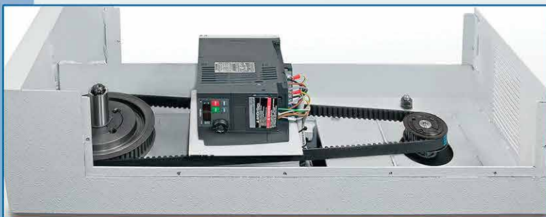
Trasmissione con variatore elettronico (Speedtronic) Modd. 13/18/22/25/30/35/40/45 • Trasmissione con variatore elettronico • Variation des vitesses par variateur électronique • Electronic speed variator • Elektronische Stufenlos
